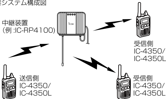
中継システム構成図
