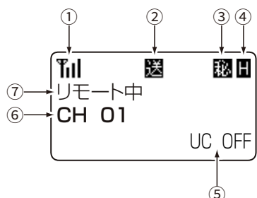
コマンドマイク(HM-206)の表示部
